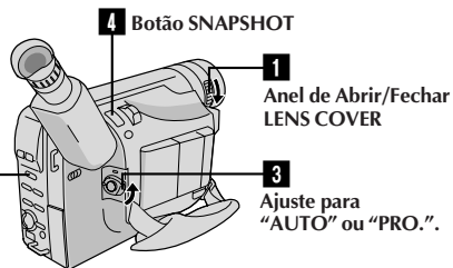
2 Ajuste-o a "D.S.C.".
